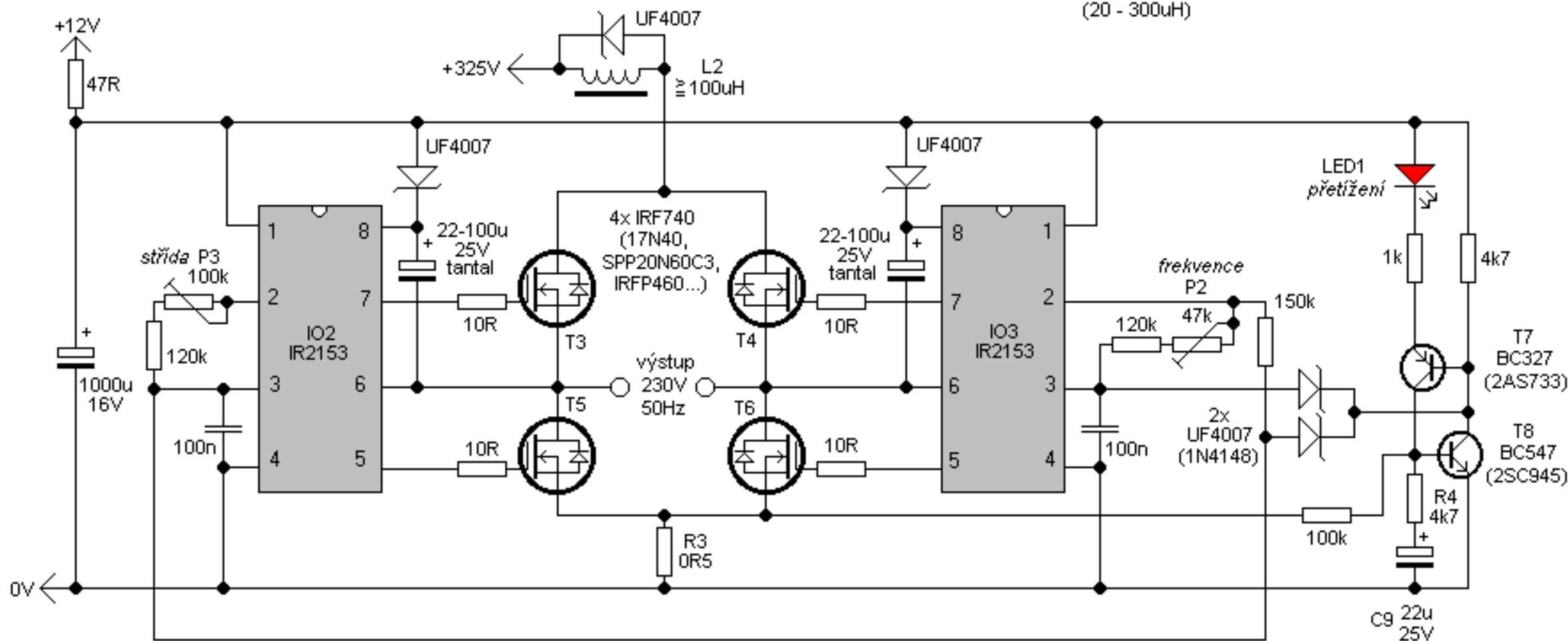
Spínaný měnič 12 / 230V s modifikovanou sinusovkou 150VA
